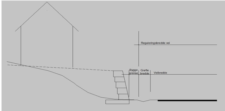
Figur 2 Plassering av forstøttningsmur som er satt opp for å øke utnyttelsen av privat tomt
